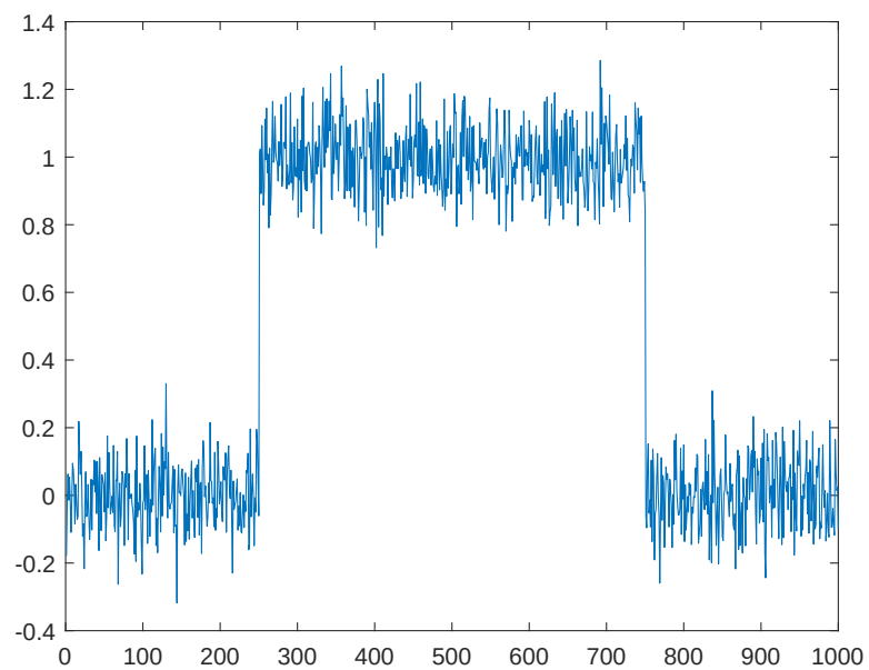
Obr. 4: Obdĺžniková funkcia s šumom
